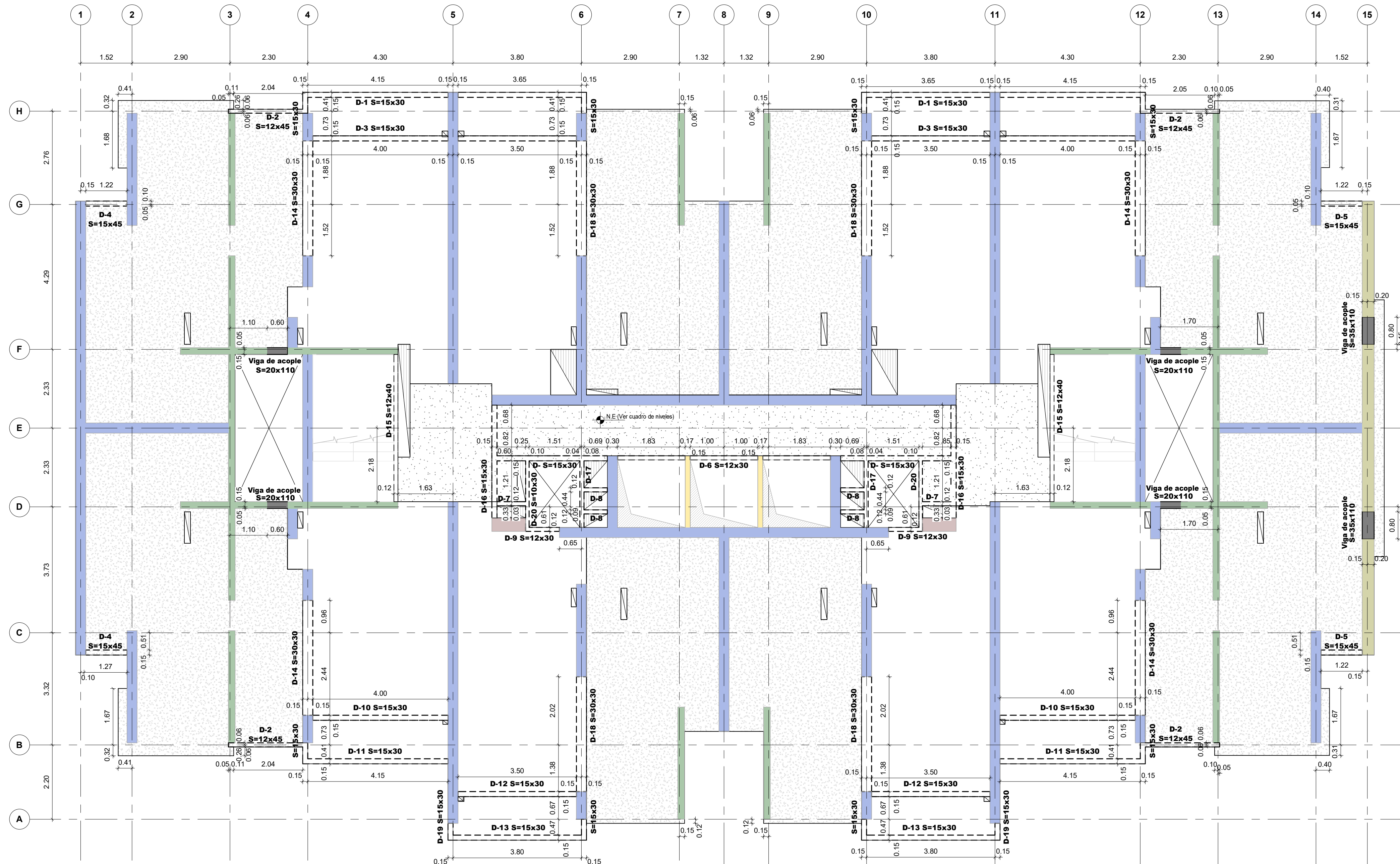
PLANTA LOCALIZACIÓN DE DINTELES PISO TIPO 3 ( PISO 23 A PISO 28 ) Escala 1 : 75
